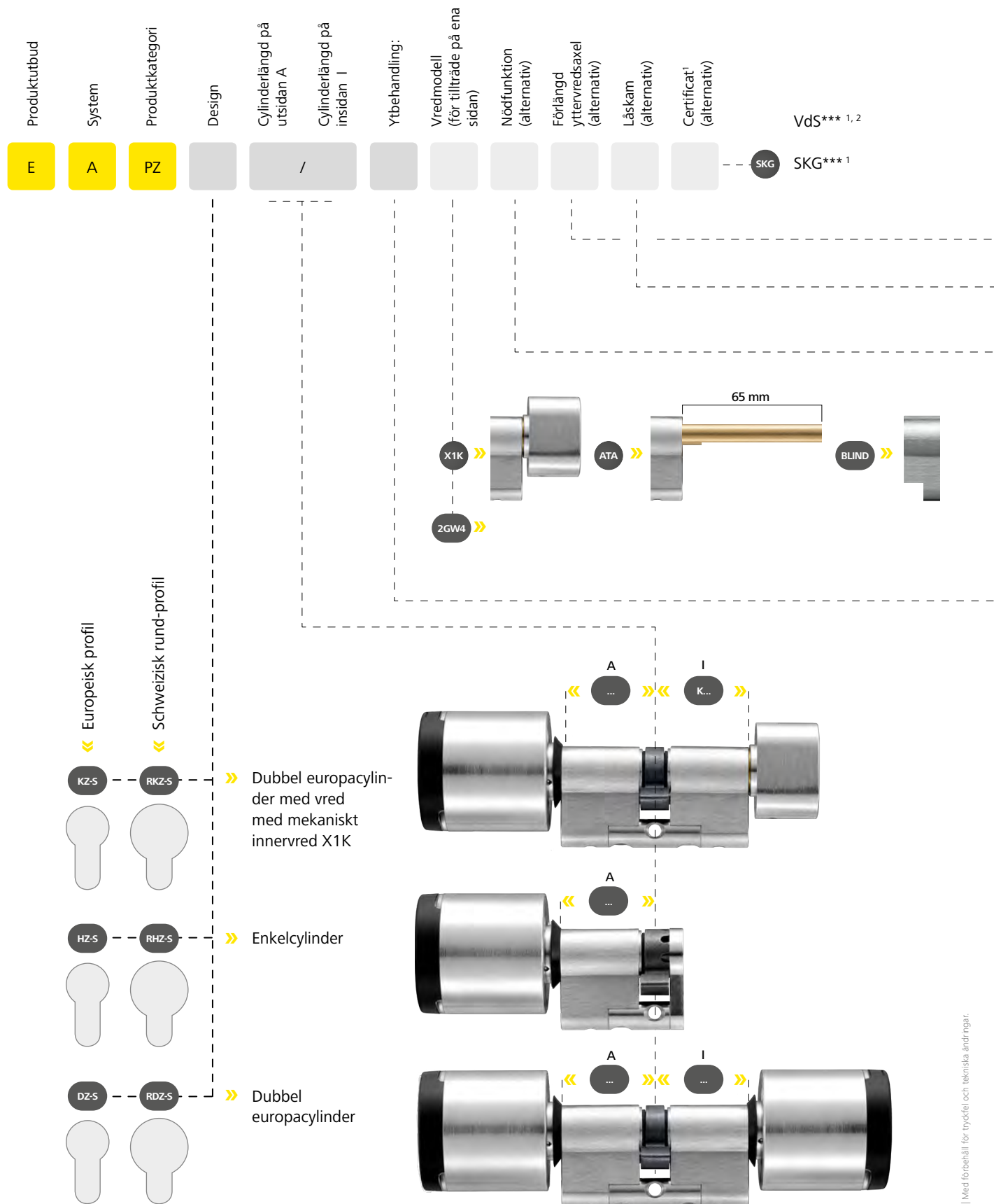
Cylinder illustrerad som europeisk profil Finns även som schweizisk rund-profil
